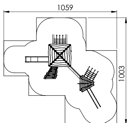
plattegrond
